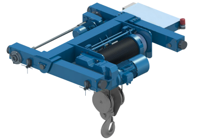
ÇİFT KİRİŞLİ VİNÇ KEDİSİ TROLLEY CRANE
