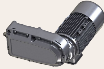
KALDIRMA MOTOR/FREN REDÜKTÖRÜ LIFT MOTOR/BRAKE GEAR
