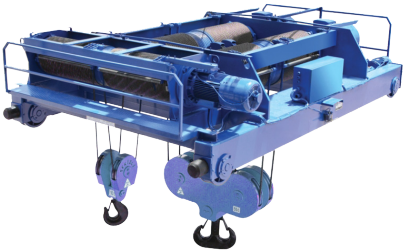
ÇİFT KİRİŞLİ VİNÇ KEDİSİ TROLLEY CRANE
