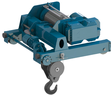
ÇİFT KİRİŞLİ VİNÇ KEDİSİ TROLLEY CRANE
